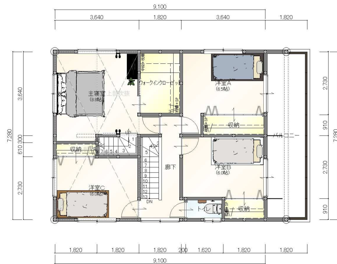
2階平面図
