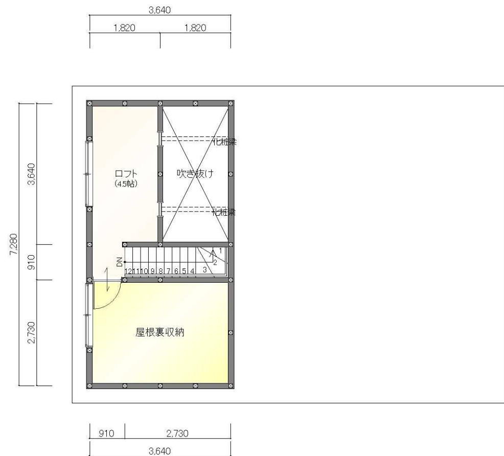
小屋平面図
