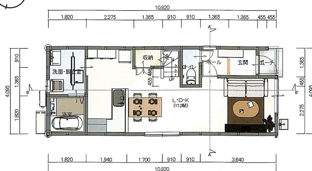
1階平面図
