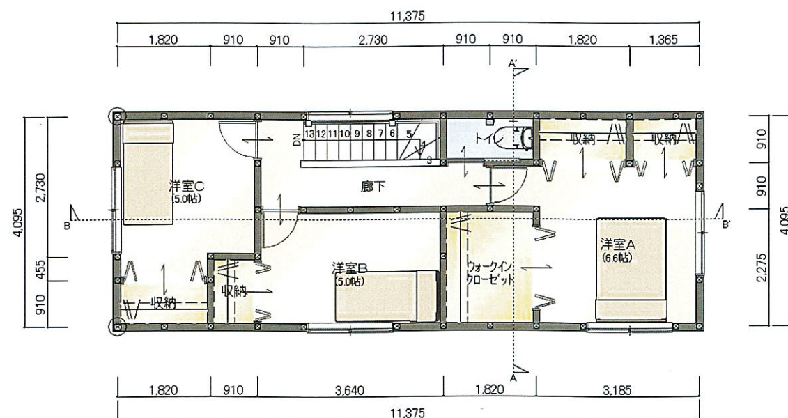
2階平面図
