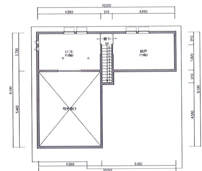
2階俯瞰図
